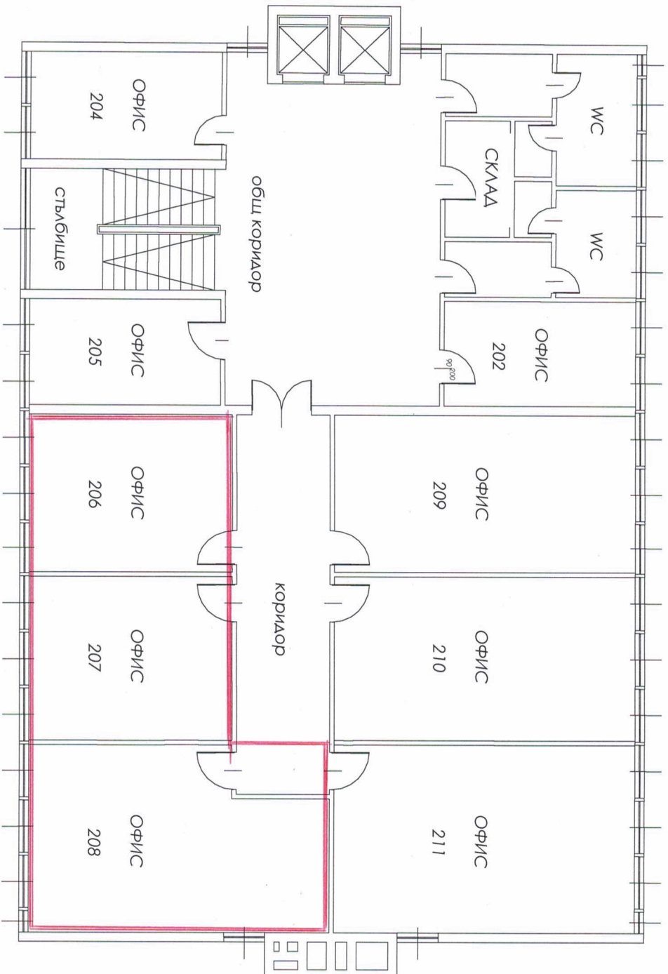
РАЗПРЕДЕЛЕНИЕ ЕТАЖ 3
